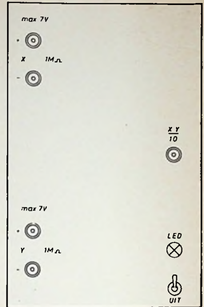
Fig. 16. Indeling van het frontpaneel van de analoge vermenigvuldiger.
